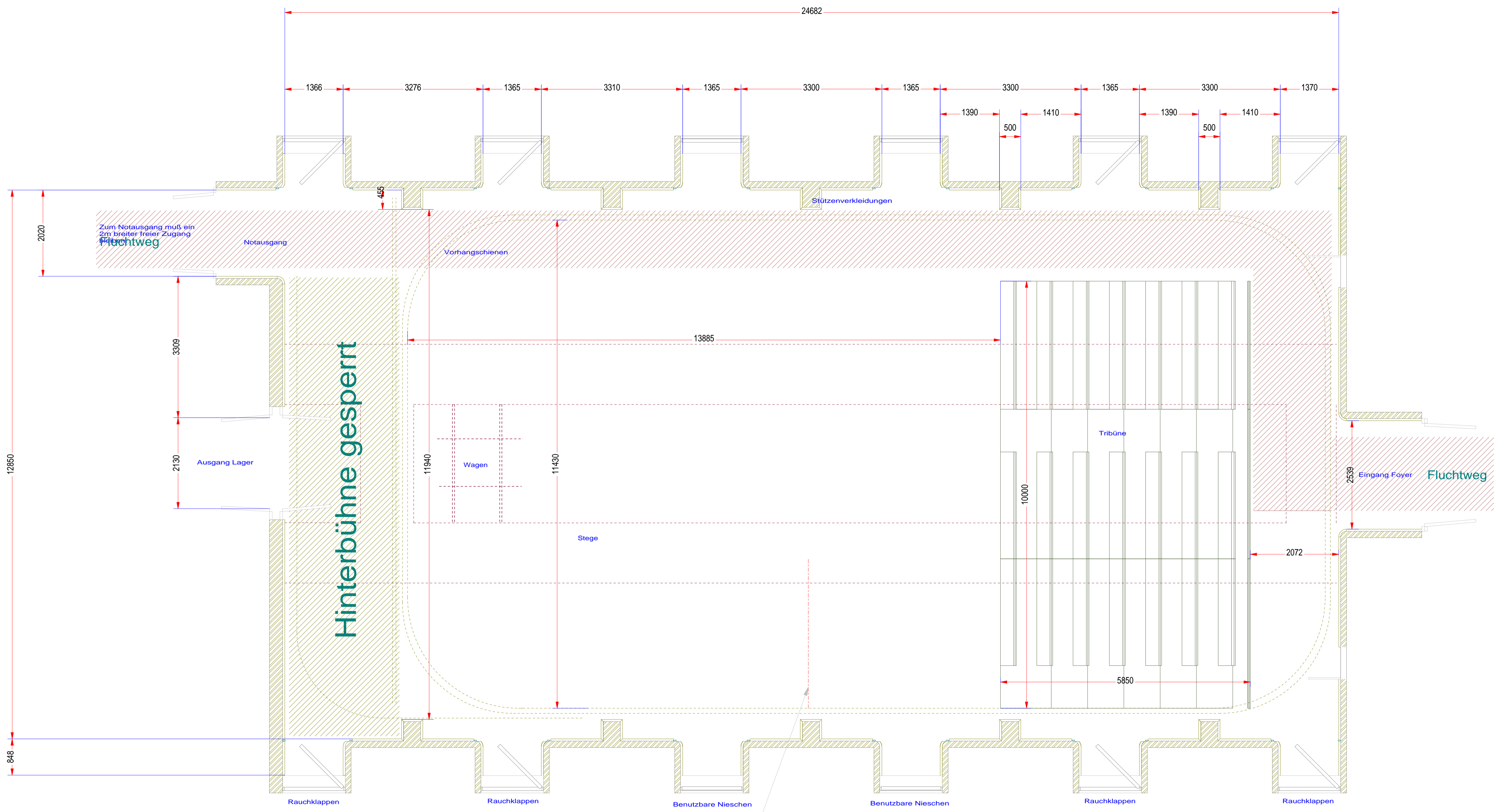
Grundriss Schnawwl
